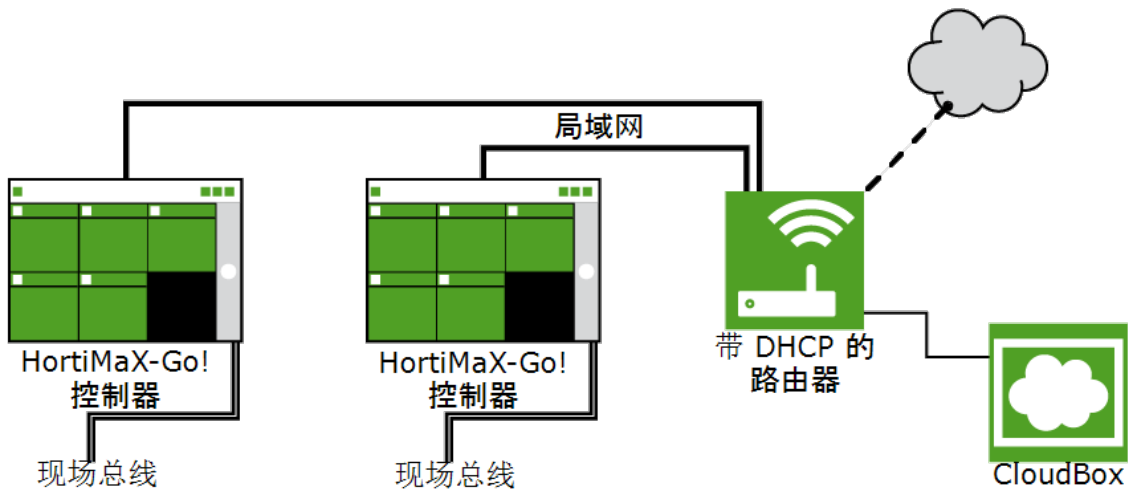
图 1-1: 网络连接图
